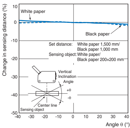
E3AS-F1500□
