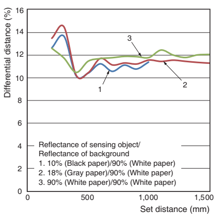
E3AS-F1500□
