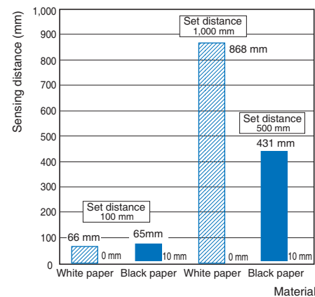
E3AS-F1000□
